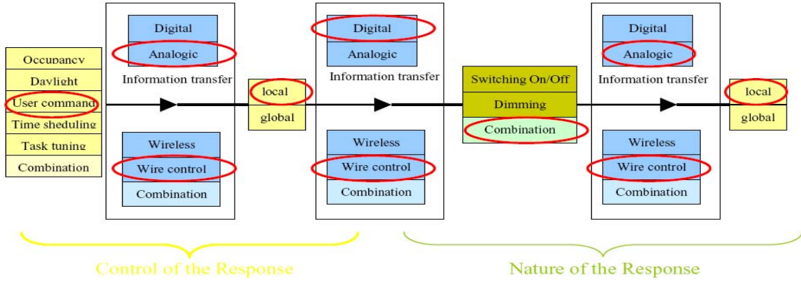
Figure10-7. TypeofcontrolinRoomG435.
